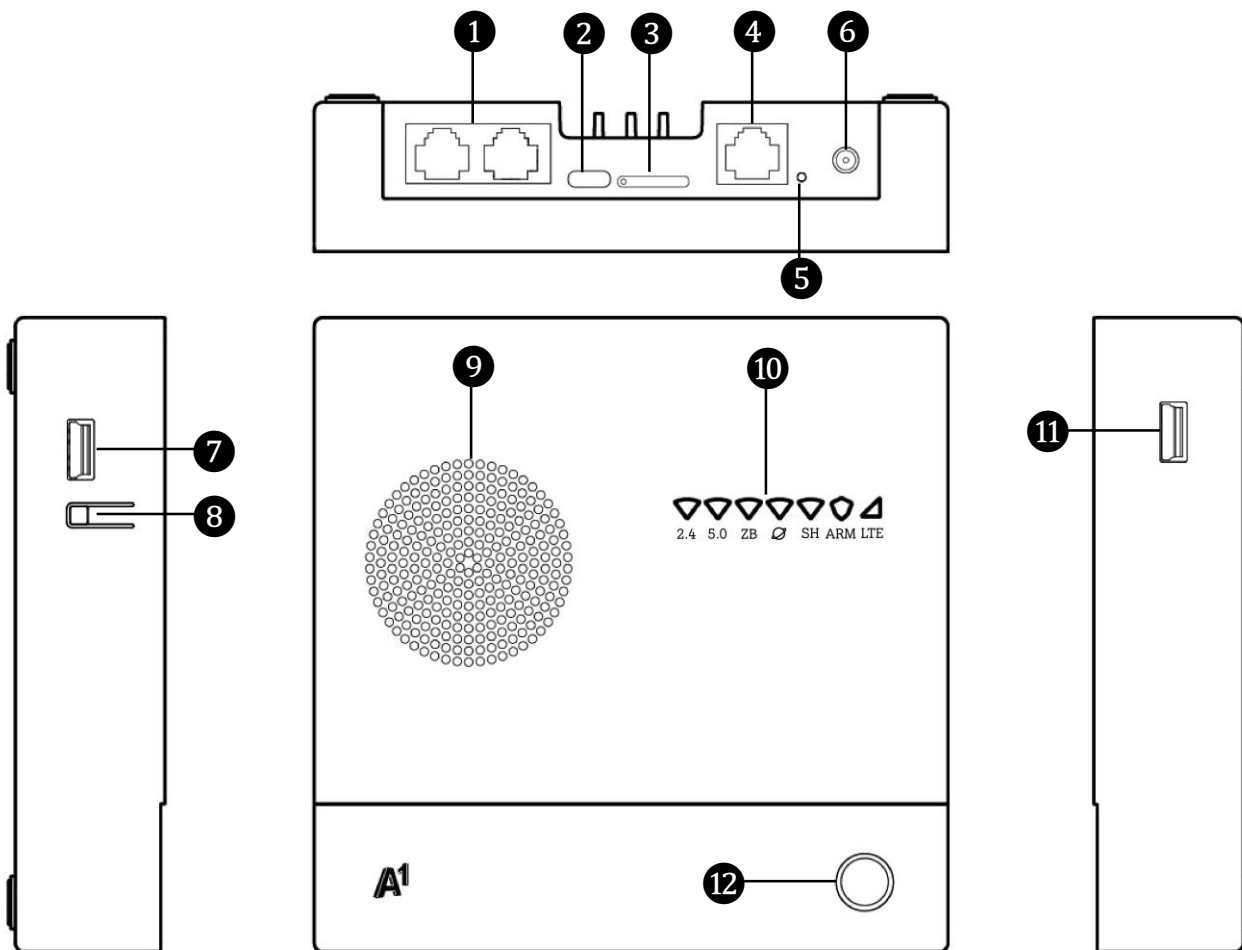
Рисунок 1 - Внешний вид
