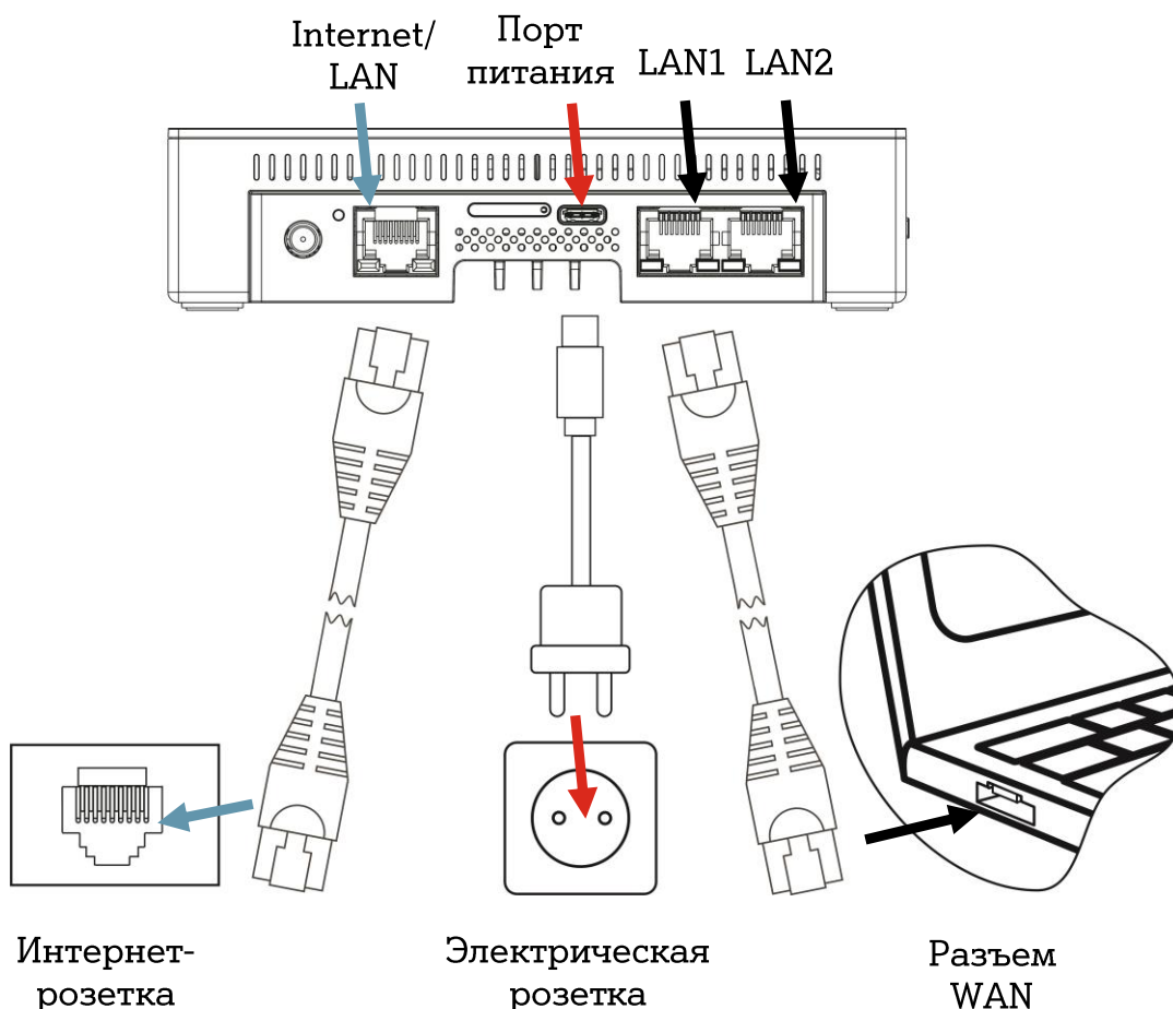
Рисунок 10 – Подсоединение к Интернет-розетке, электрической розетке и ноутбуку
