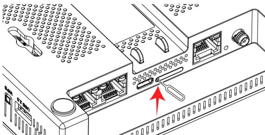
Рисунок 14 - Извлечение держателя SIM-карты из корпуса
