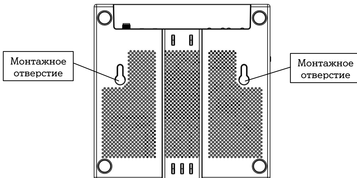
Рисунок 12 – Отверстия для крепления на стену
