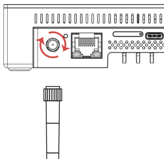
Рисунок 13 – Прикручивание наружной антенны
